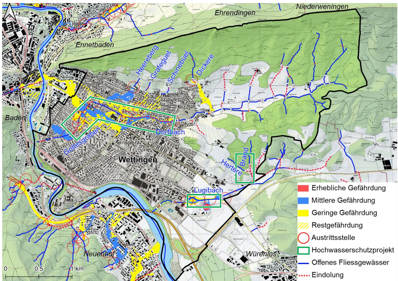
Abbildung 2 Gefahrenkartierung Wettingen
