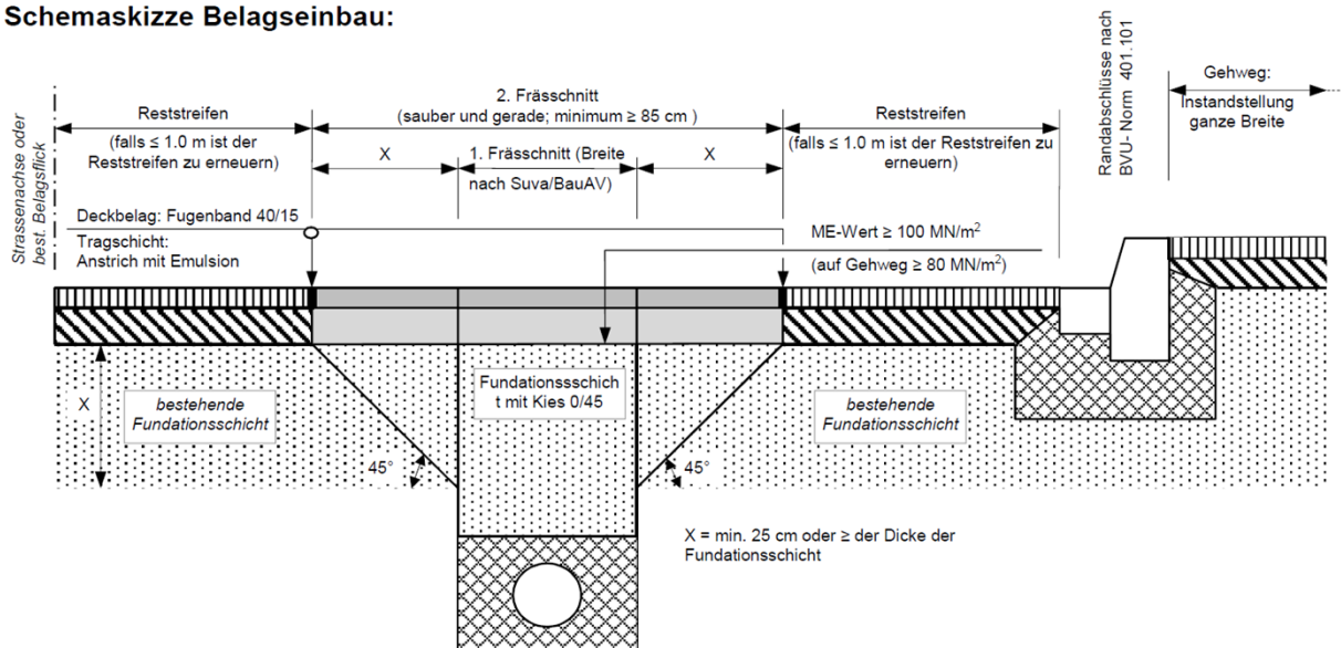
Schemaskizze Belagseinbau:
