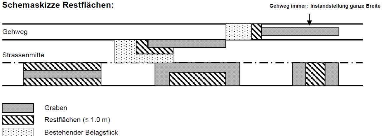
Schemaskizze Restflächen:
