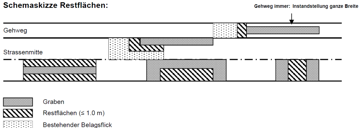
Schemaskizze Restflächen:
