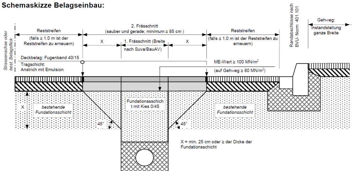
Schemaskizze Belagseinbau:
